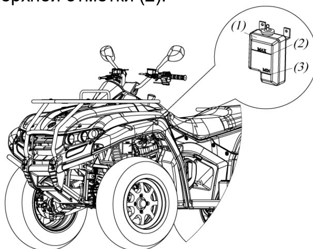
Рисунок 17 – Расширительный бачок
